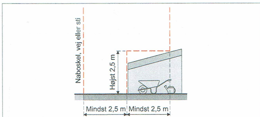
FIGUR 37. Maksimal højde for bygninger i tilknytning til sommerhuse, der kan placeres inden for en afstand af 2,50 meter og 5,0 meter fra skel mod nabo, vej eller sti for overholdelse af byggeretten.
